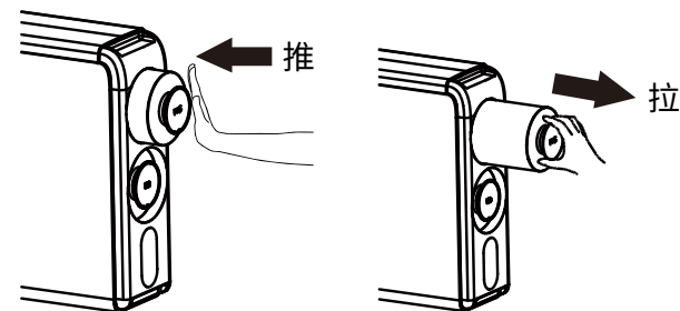
(3) 選擇需要更換的濾心向內推，聽到「喀」一聲，即可將濾心拉出
