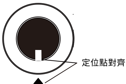
(4) 換上相同規格的濾心，將濾瓶插入到對應的濾瓶孔內，濾瓶蓋定位點與面板定位點對齊
